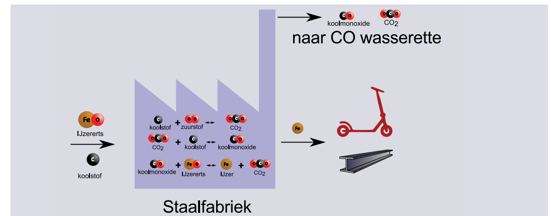
Figuur 4: Zo wordt ijzer uit ijzererts gemaakt. Als de koolmonoxide schoongemaakt kan worden in de ‘wasserette’, dan kan schone CO daarna benut worden als grondstof in de chemie.”
