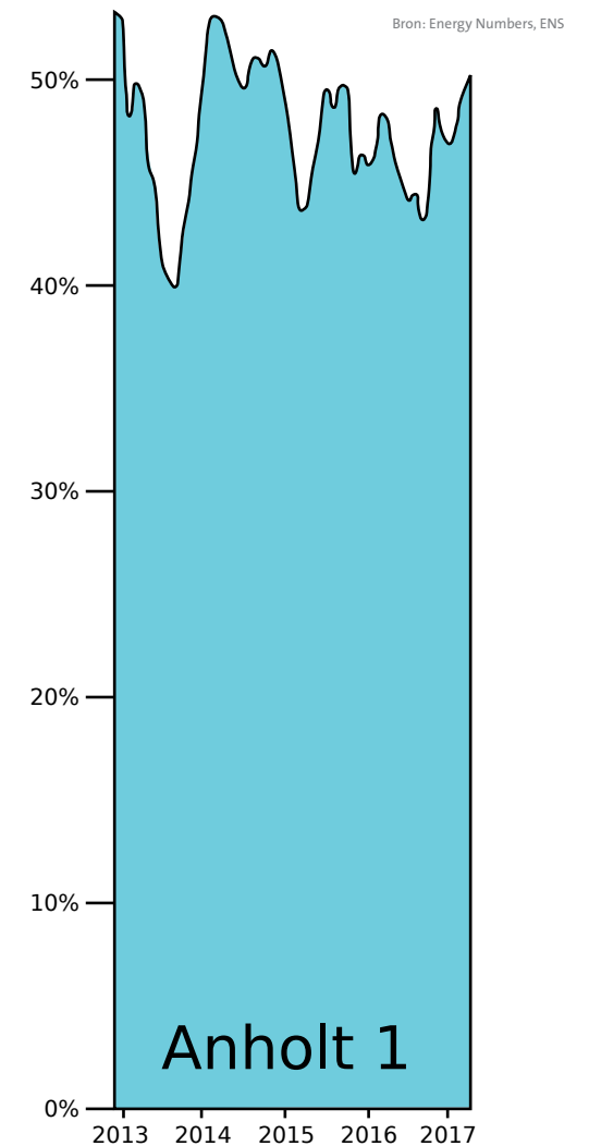
Figuur 14: In het Deense windpark Anholt 1 wordt al regelmatig een capaciteitsfactor van 50% gehaald.
