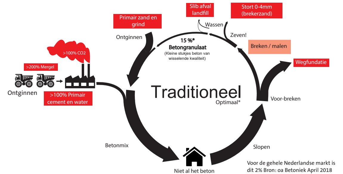
Figuur 10: De huidige manier van beton maken zorgt voor veel \text{CO}_2 -uitstoot.
